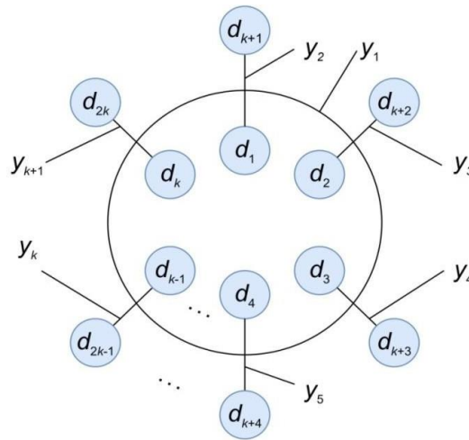
Рисунок 1 – Гиперграф H(D,Y)
